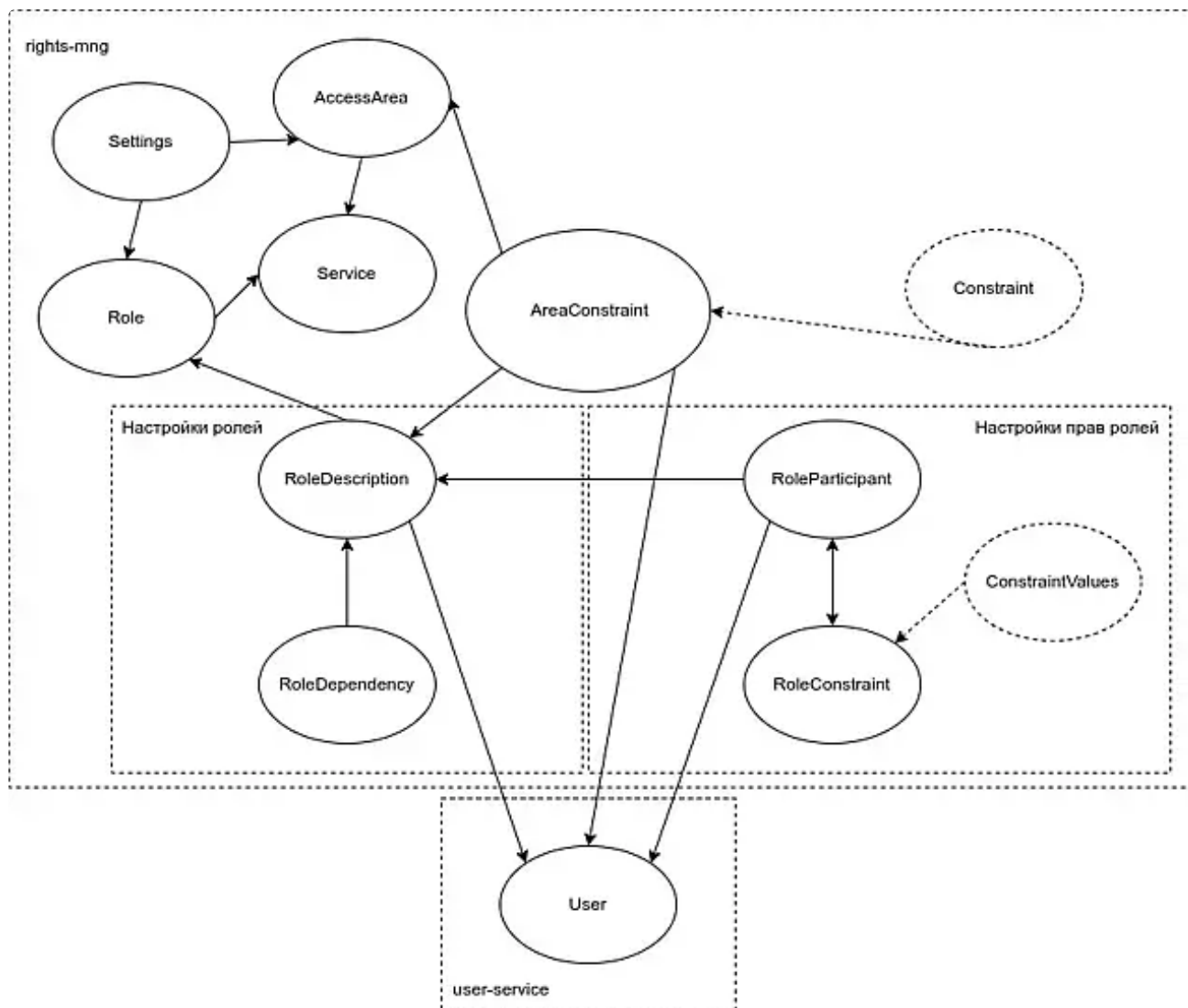
Рис. 2. Схема сущностей системы прав на сервисе rights-mng
