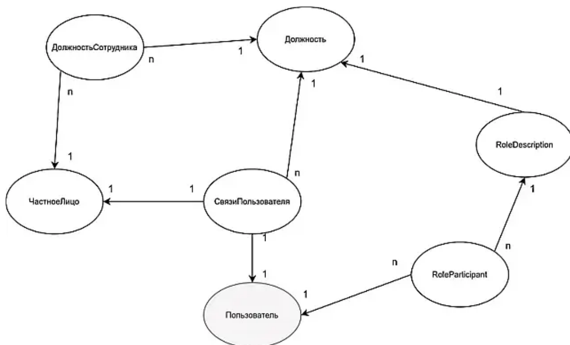
Рис. 5. Схема связи ролей с должностями на основном сервисе
