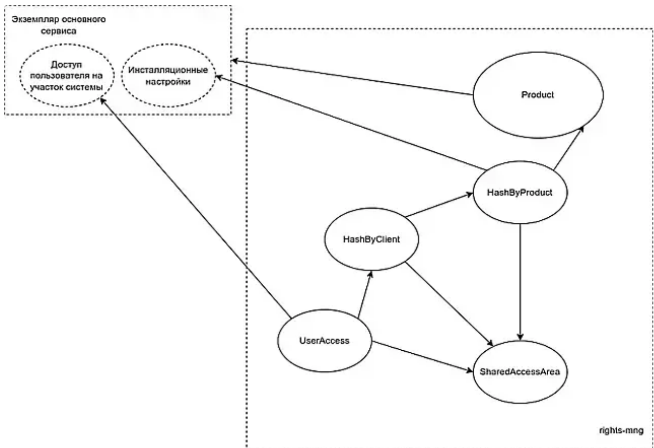
Рис. 3. Схема сущностей проксируемых прав с основного сервиса через rights-mng
