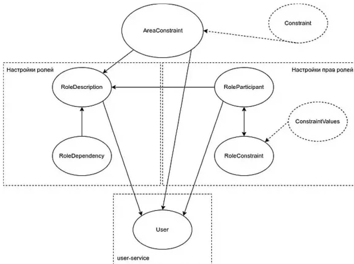
Рис. 1. Схема сущностей на сервисе с локальной системой прав
